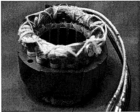
Thermal Cutout
